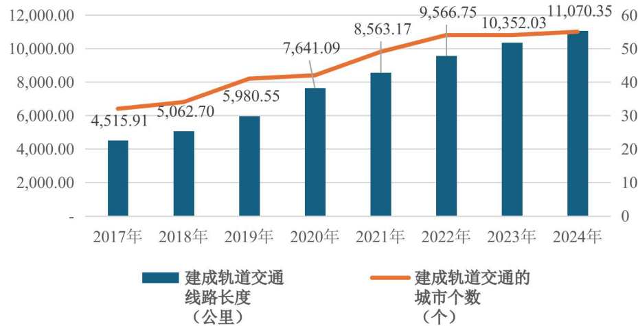
全国城市轨道交通建设情况
