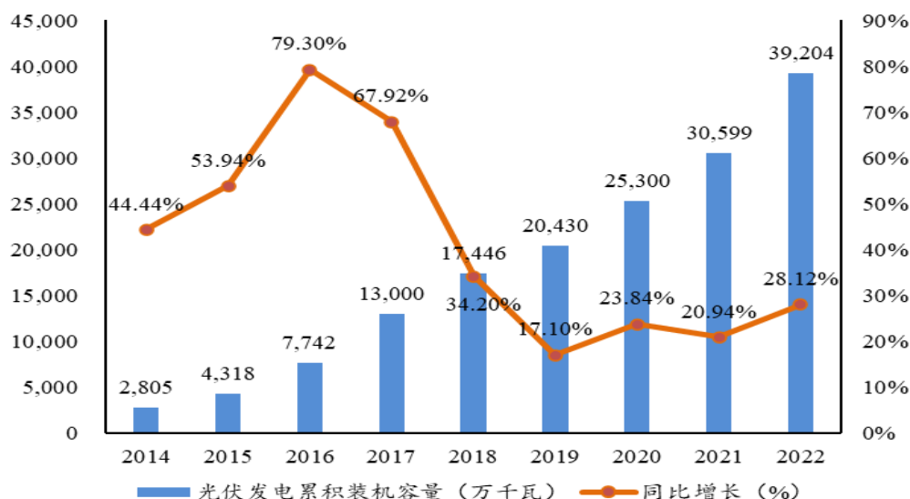
2014-2022 年全国光伏发电累计容量及增长率
