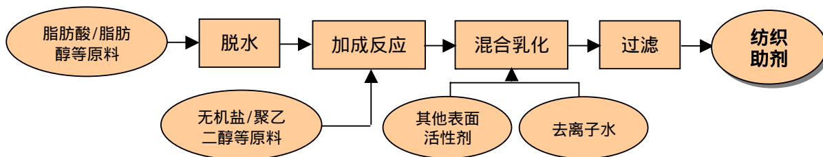
纺织助剂生产工艺流程图
