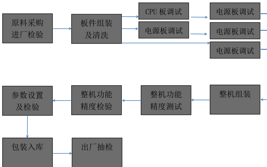
④高压计量产品工艺流程图：
