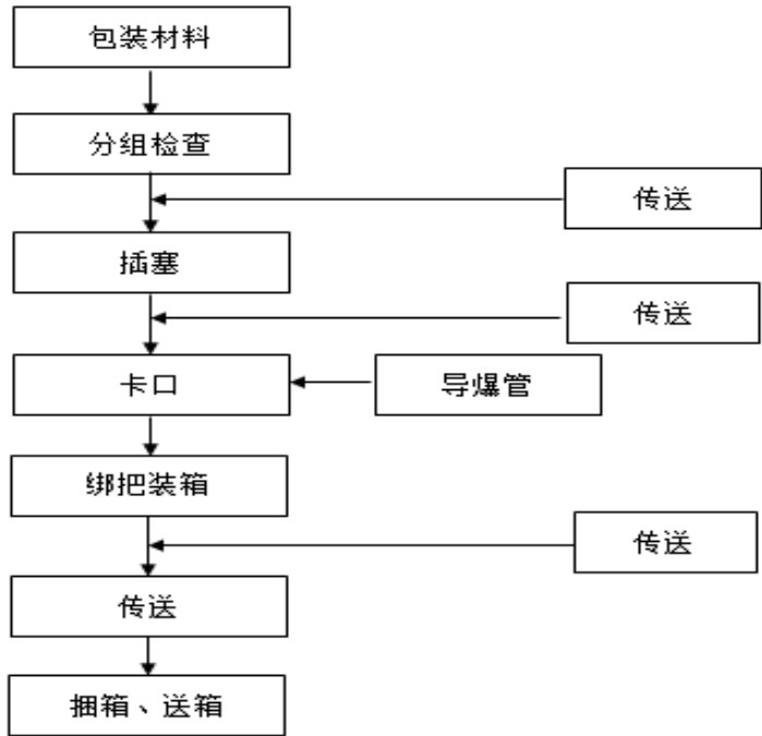
2、爆破服务工艺流程图
