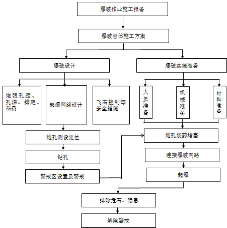
2、爆破服务工艺流程图
