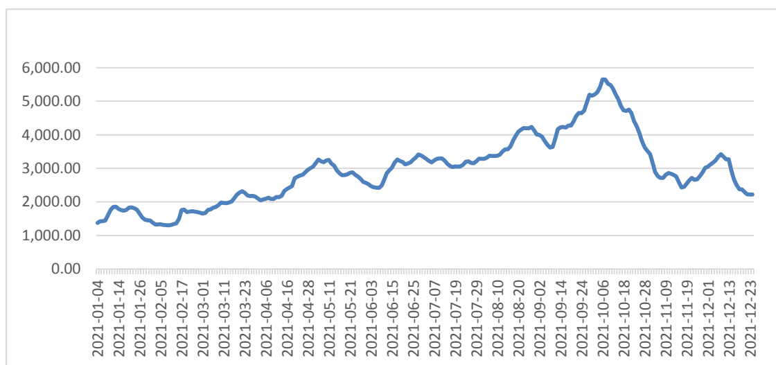
图 4-1：2021 年波罗的海干散货指数 (BDI)
