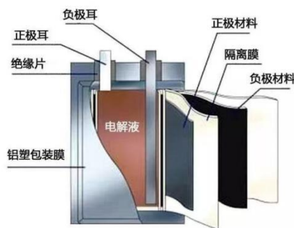
图：锂电池结构示意图
