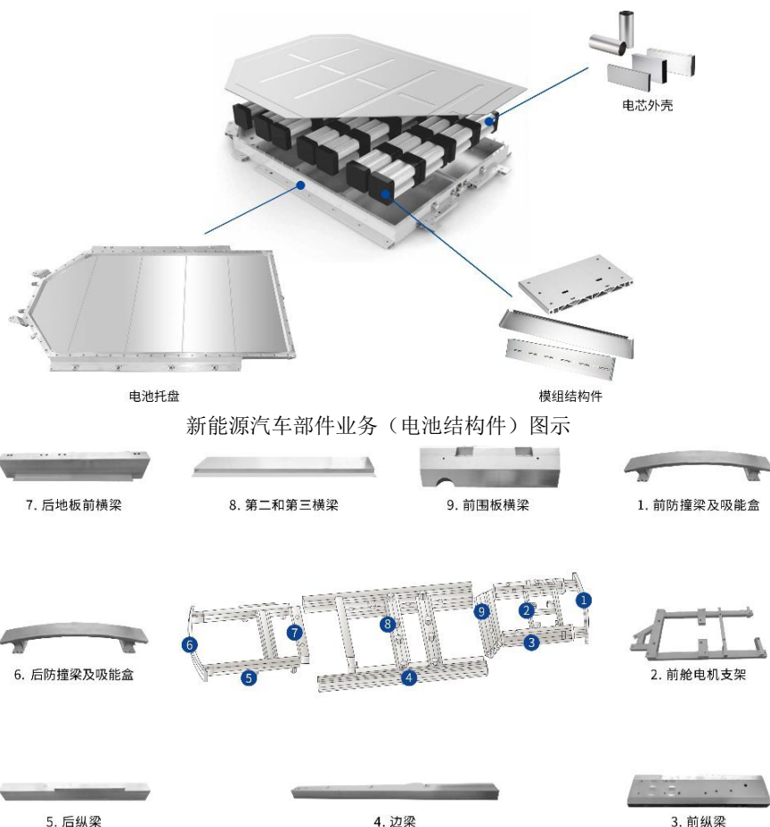
新能源汽车部件业务（车身结构件）图示
