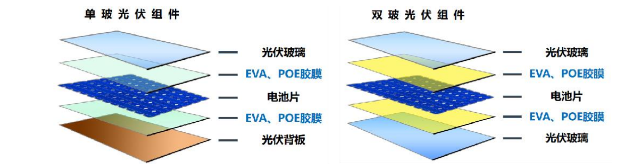
图：单/双玻组件结构示意图
