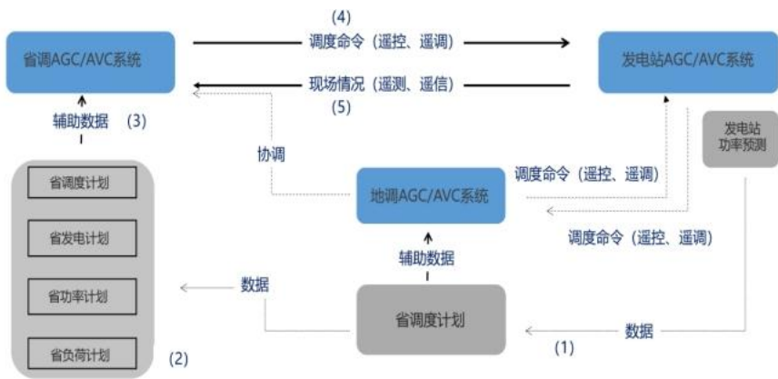
图 7：自动发电控制系统和自动电压控制系统的控制过程图
