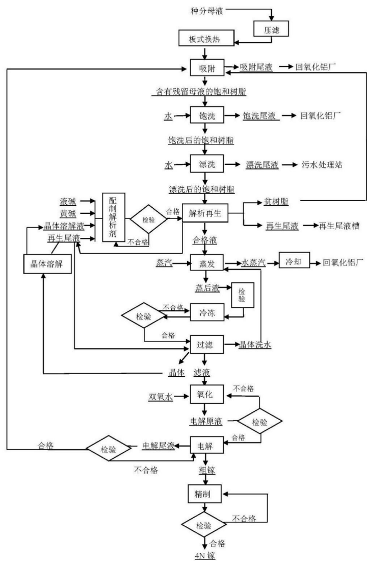
三门峡铝业金属镓碱法生产工艺流程图
