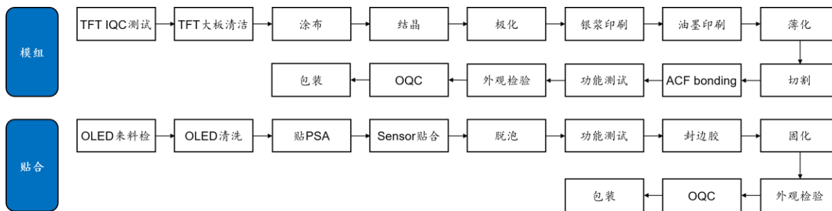
(3) 超声波指纹识别模组工艺流程图
