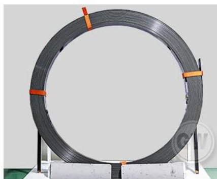
风电碳梁
