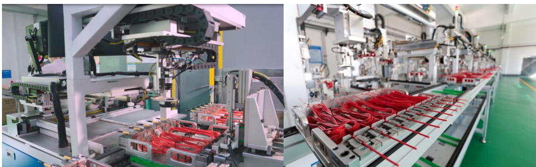
图十 电子雷管生产线
