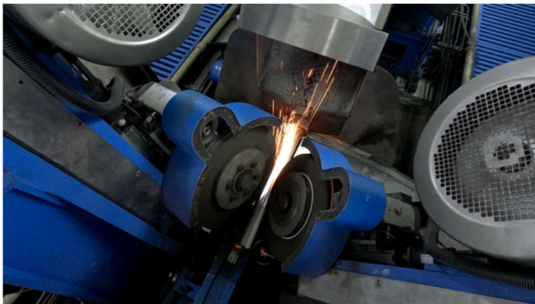
图 11：焊轨基地个性化钢轨廓形预打磨加工设备
