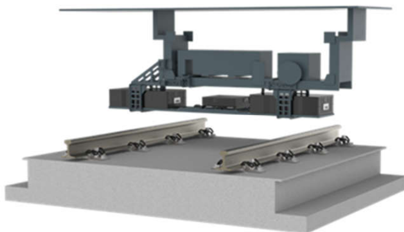
图 9: 车载式高速钢轨廓形测量仪
