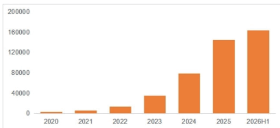
图 11：2021-2026 年上半年中国新型储能累计装机规模（兆瓦）
