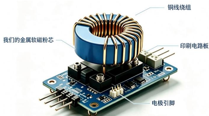
金属软磁粉芯集成至客户终端产品的结构图解
