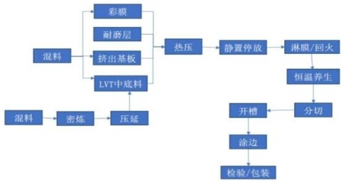
(3) AB 贴合热压生产工艺流程图
