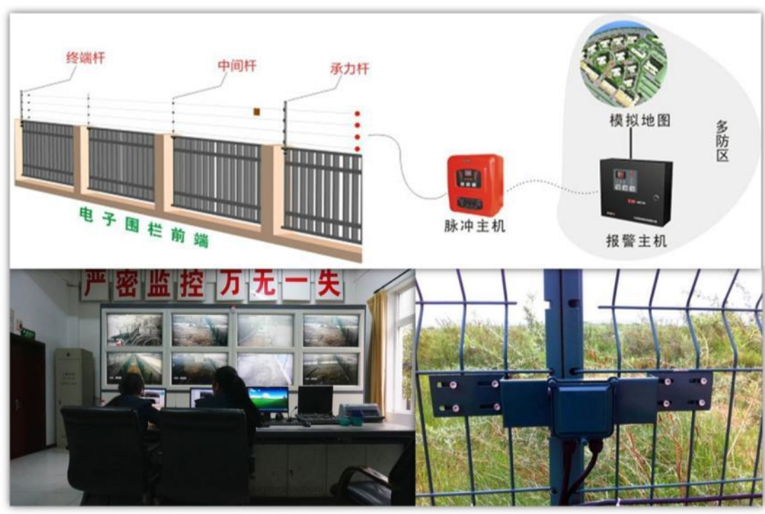
通宝莱智能光电防入侵系统示意图
