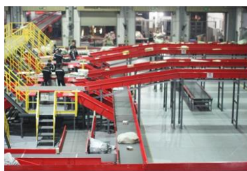
图6.25 中转场配备的自动分拣机
