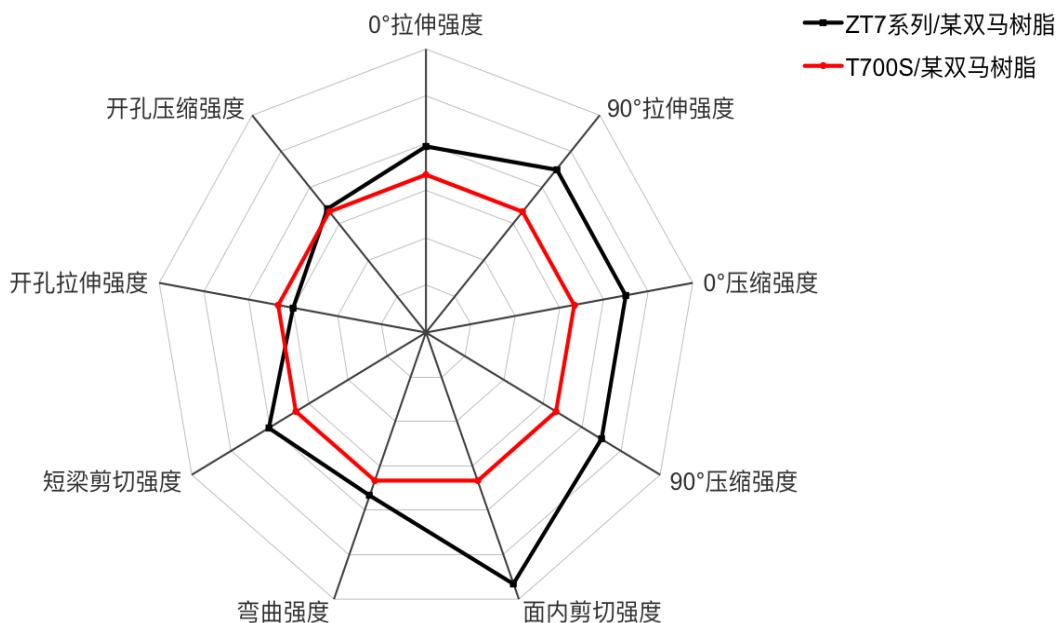
图6-26： ZT7系列牌号与日本东丽T700S级碳纤维生产的复合材料相关性能指标对比图
