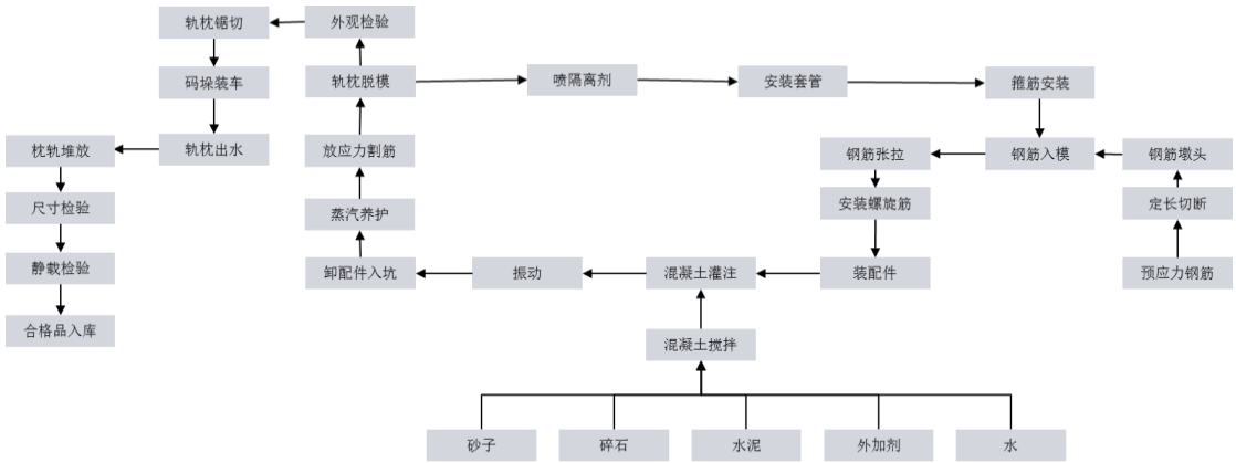
② 轨枕生产工艺流程图
