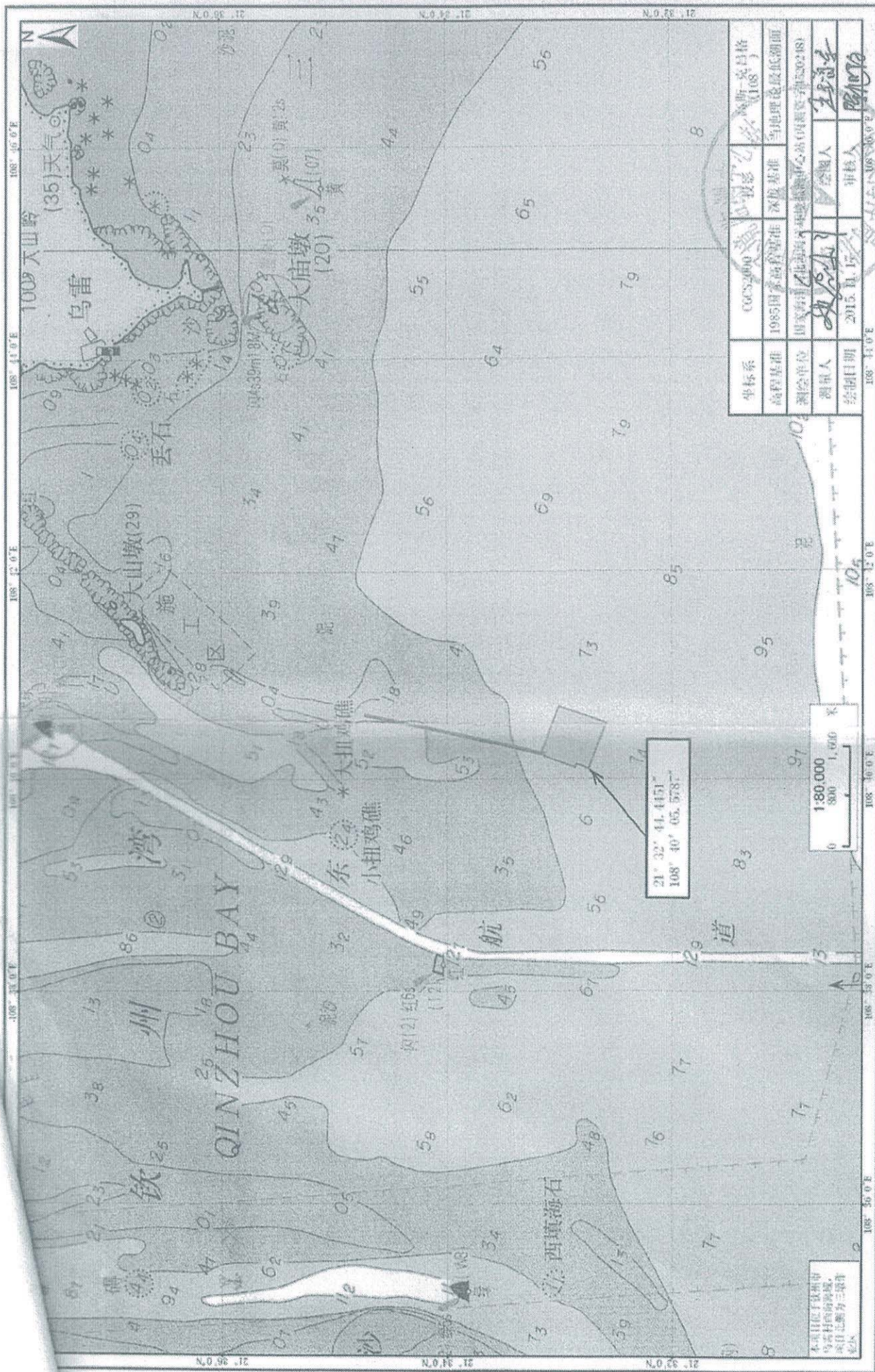
北部湾钦州30万吨级油码头工程宗海位置图
