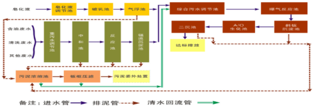
污水处理工艺流程图:
