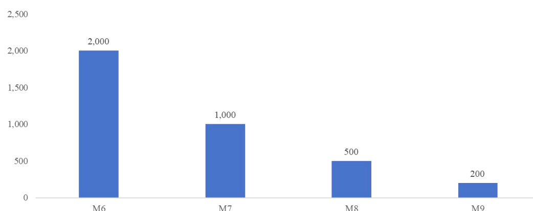
图：主流 PCB 材料单板单针可加工孔数
