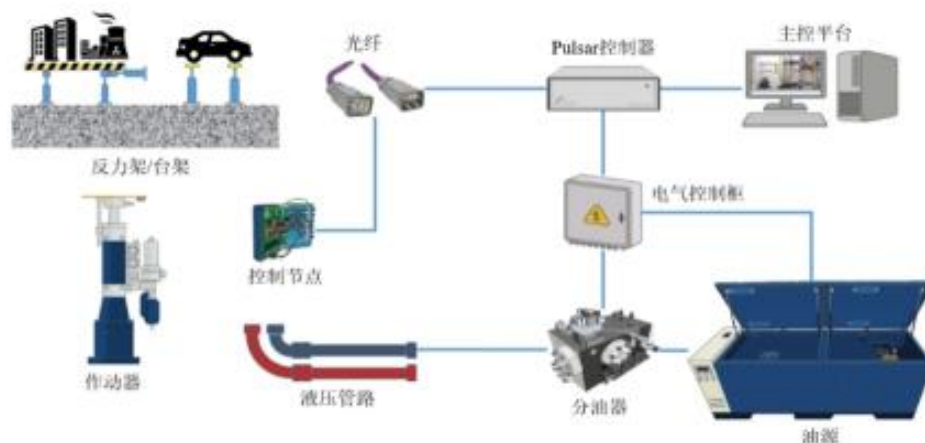
伺服液压测试设备组成图示
